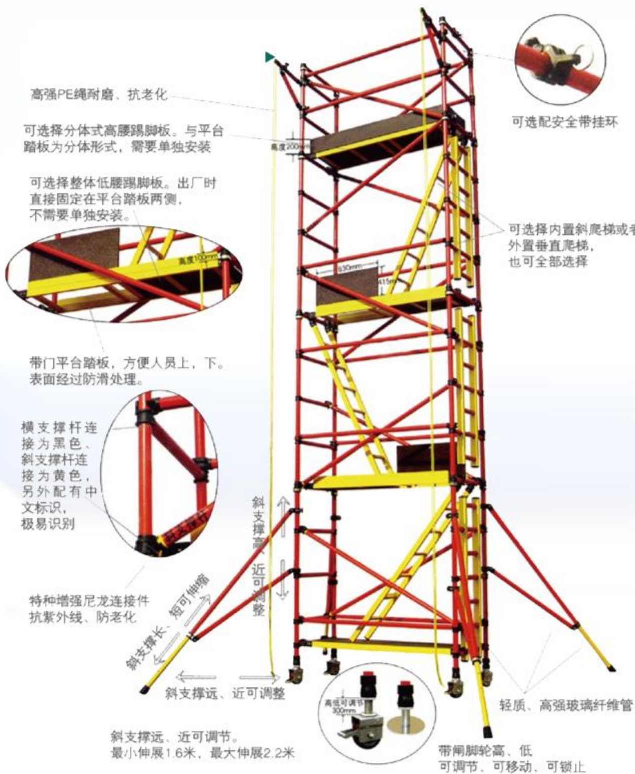
绝缘脚手架
