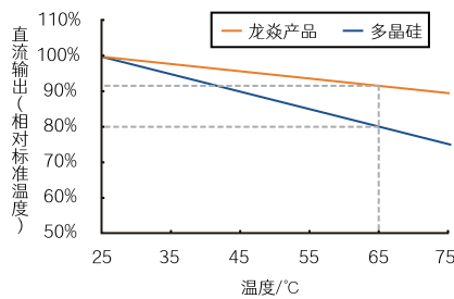
不同温度下发电性能对比
