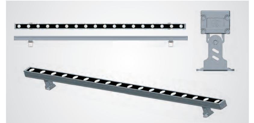
产品型号: YJ-普通私模漏水款 灯具尺寸: 31*25*1000MM 光源: Cree/Osram/Epistar/Bridgelux 额定功率: 18W/24W 输入电压: DC24V 灯具材质: 6063航空拉伸铝 半结构防水灯具 光色: 1800K-7500K, 全系单色光, RGB, RGBW 表面处理: 户外等级喷涂, 常规UV 10年保护。/硬质阳极氧化 IP等级: IP65
