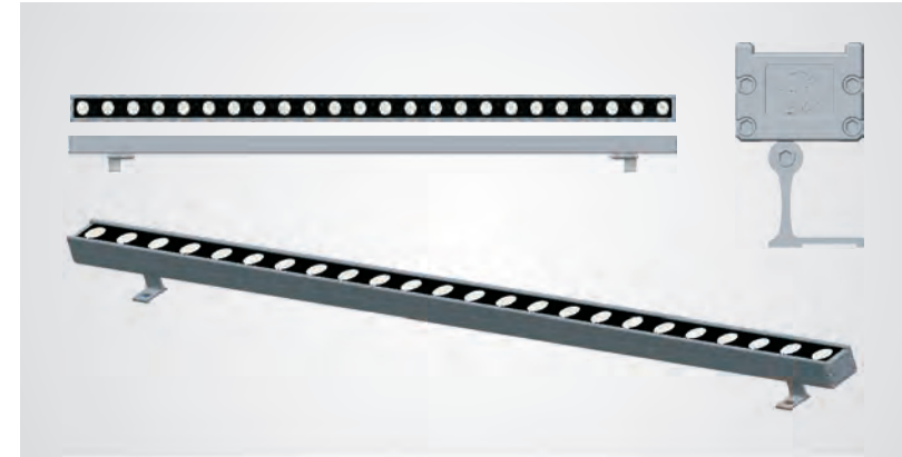
产品型号: YJ-FS036 灯具尺寸: 37.5*29*1000MM 光源: Cree/Osram/Epistar/Bridgelux 额定功率: 18W/24W/36W 输入电压: DC24V 灯具材质: 6063航空拉伸铝 纯结构防水灯具 光色: 1800K-7500K, 全系单色光, RGB, RGBW 表面处理: 户外等级喷涂, 常规UV 10年保护。/硬质阳极氧化 IP等级: IP65
