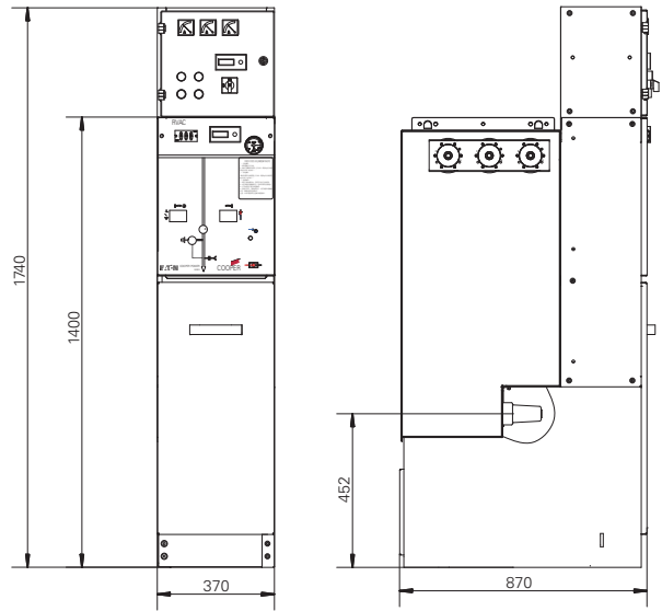
T 柜
