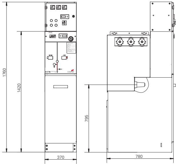
K 柜
