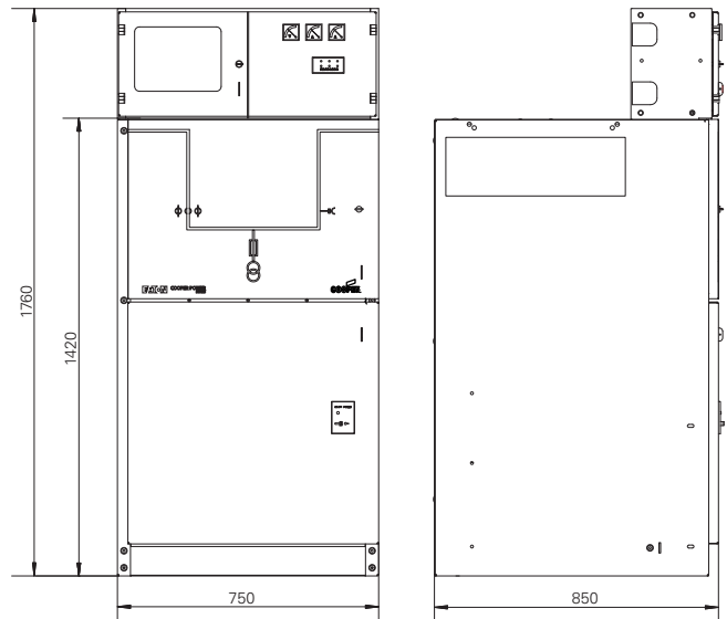
M 柜
