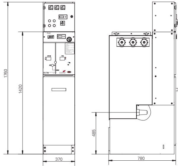
T 柜
