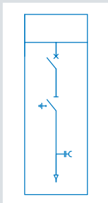
断路器柜 “V” & “CB”
