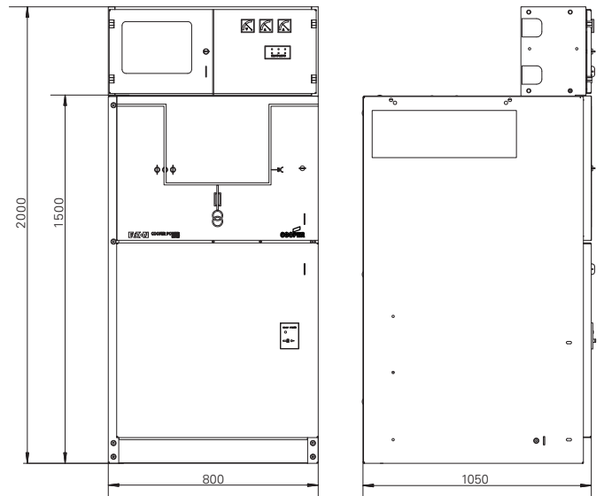
M 柜
