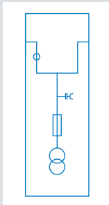
计量柜 “M”
