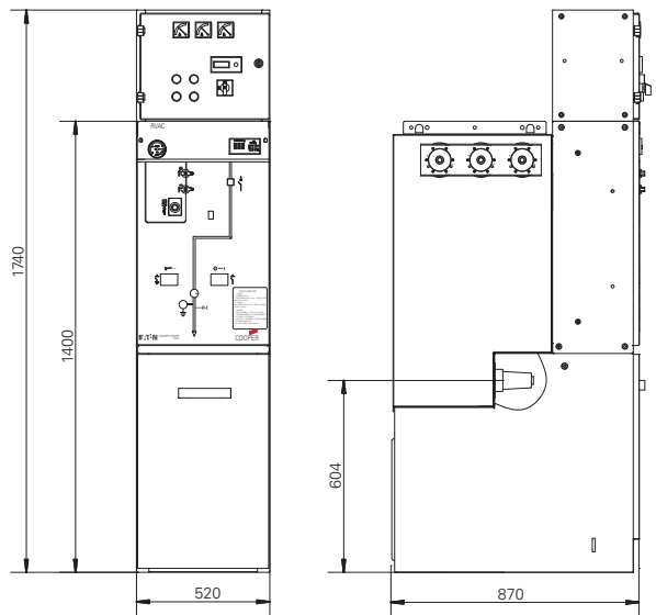
V 柜
